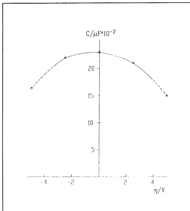
Slika 3: Kapacitivnost komercialnega elektrokemijskega kondenzatorja v odvisnosti od prenapetosti, določena iz frekvenčnega odziva v območju 10^{-1} do 10^4 Hz.
