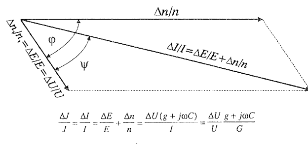
Slika 3: Kazalčni diagram izmeničnih signalov v NIN strukturi
