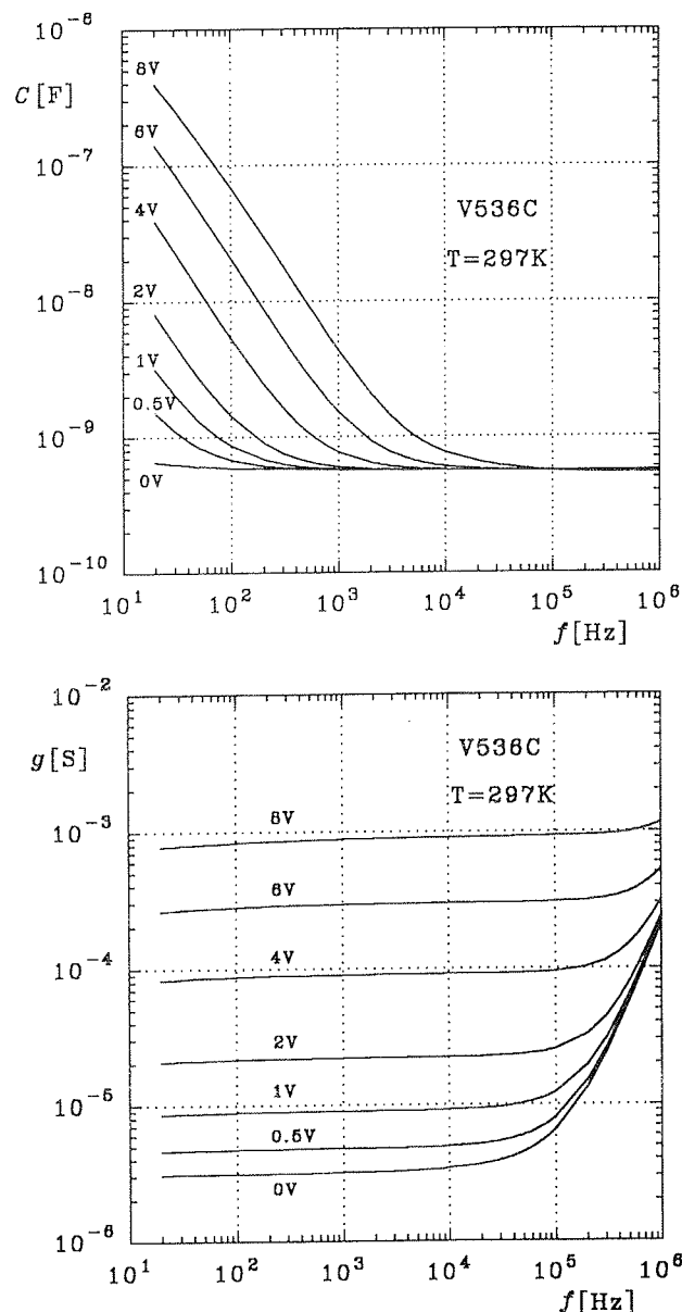
Slika 1: Izmerjena diferencialna kapacitivnost in ohmska prevodnost NIN strukture v odvisnosti od enosmerne prednapetosti in od frekvence
