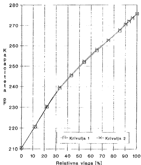
Slika 3: Sprememba kapacitivnosti senzorja vlage v odvisnosti od relativne vlažnosti. Krivulja 1 je bila posneta med naraščanjem vlage, krivulja 2 med njenim padanjem. Temperatura je bila konstantna 23°C.
