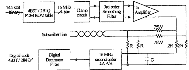
Figure 3. U-interface analog front-end anno 1987
