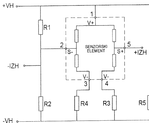
Slika 3 Kompenzacija tokovno napajanega senzorjskega mostiča
