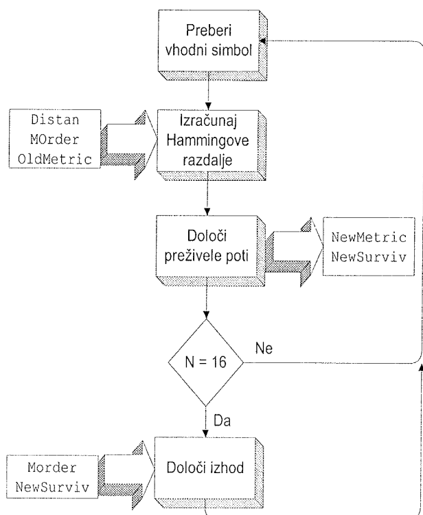
Slika 3: Viterbijev dekodirnik
