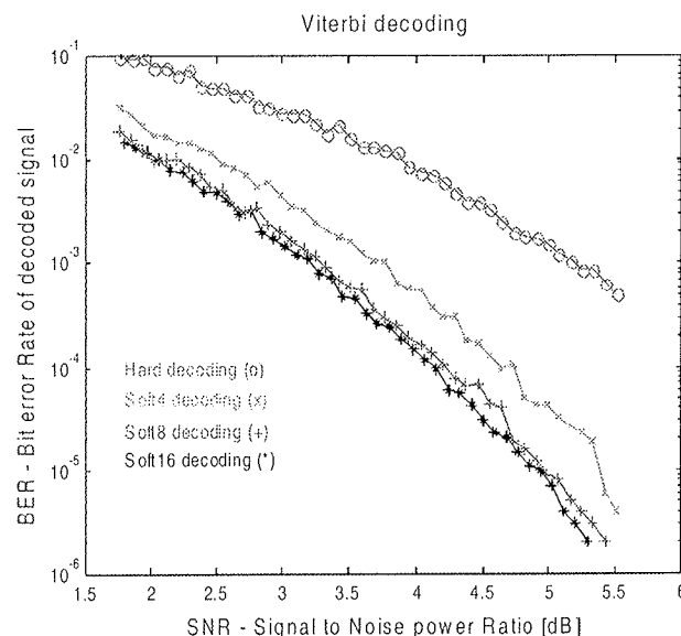
Slika 4: BER diagram za različne Viterbijske dekodirnike
