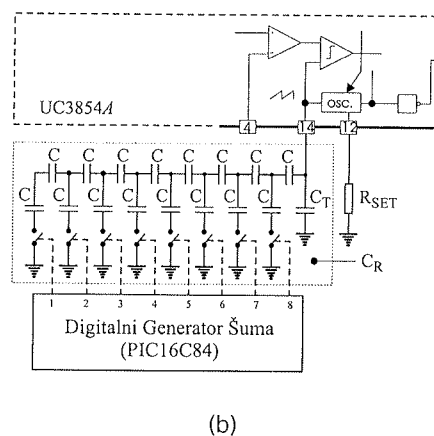
Slika 5: (a) Krmilna enota usmernika, (b) Princip naključne modulacije: mreža kondenzatorjev in digitalni generator šuma.
