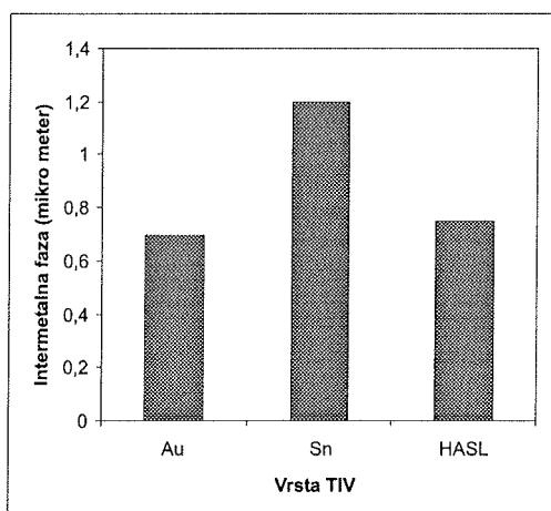
Slika 5: Debeline intermetalnih plasti glede na vrsto TIV (Au – zlatena; Sn – kositrena; HASL – Hot Air Solder Leveling)
