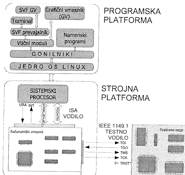
Slika 3: Strojna ter programska struktura projekta EBS
