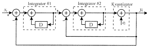
Slika 2: \Sigma\Delta modulator II. stopnje
