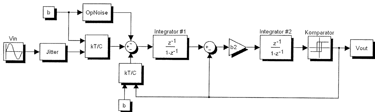
Slika 3: Blokovni diagram SC \Sigma\Delta modulatorja II. stopnje v SIMULINK-u
