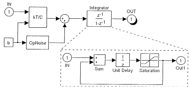
Slika 4: Model šumnega integratorja
