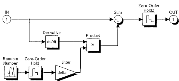
Slika 10: Modeliranje podrhtavanja vhodnega signala
