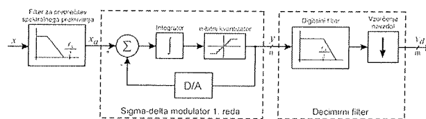
Slika 1: Blokovni diagram A/D pretvornika s \Sigma\Delta modulatorjem
