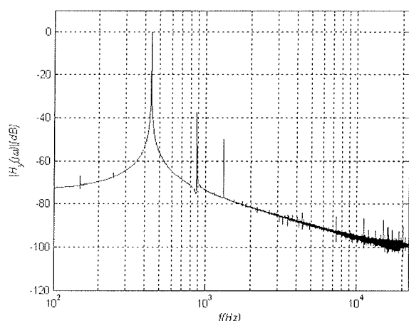
Slika 6: Frekvenčni spekter predojačevalnika s tranzistorjem na poljski učinek
