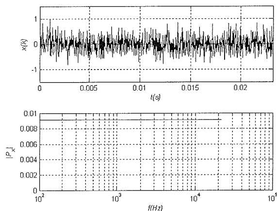
Slika 2: Časovni potek signala belega šuma x(k) in spekter moči |P_x(j\omega)|
