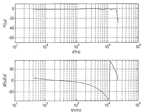
Slika 3: Amplitudni in fazni frekvenčni odziv merilnega sistema
