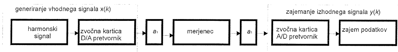
Slika 1: Blokovna shema merilnega sistema za določitev frekvenčnega spektra
