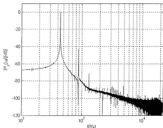
Slika 7: Frekvenčni spekter predojačevalnika z elektronko
