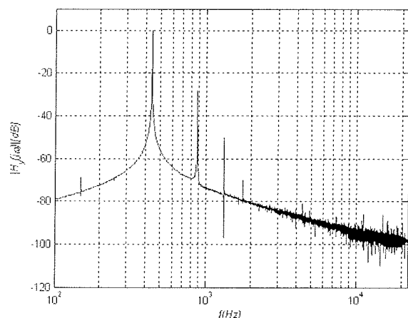
Slika 5: Frekvenčni spekter predojačevalnika z bipolarnim tranzistorjem
